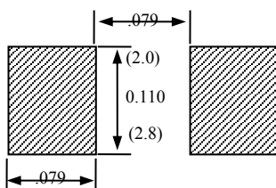
DO-214AC (SMA)
