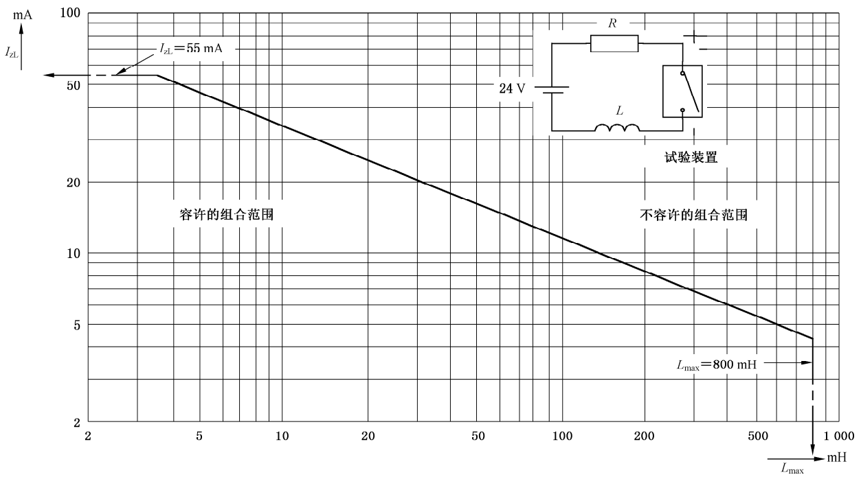
图 G.6 在乙醚蒸气和氧混合成的最易燃气体中电感电路上测得的最大容许电流 I_{zc} 和电感 L_{max} 的函数关系
