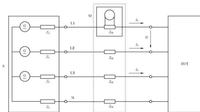
图 A.1 单相设备测量电路
